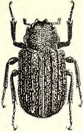
Abb. 6: Habitusbild von Paramaechidius heterosquamosus (Heller) (nach Heller)
